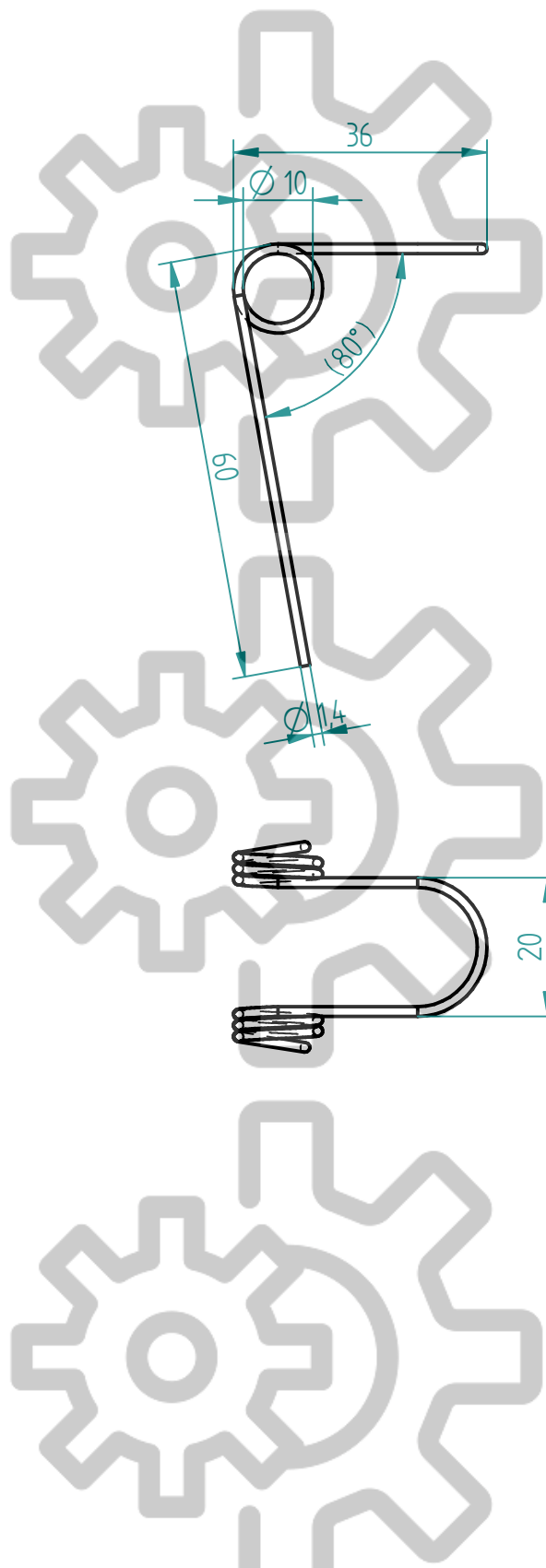
Doppelschenkel-Sicherungsfeder nach DIN 2194
